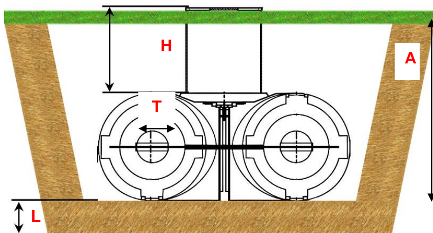
Imagen 2. Medidas de la zanja de instalación
