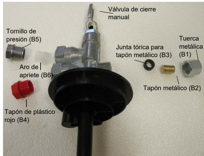
Sistema de aspiración de gasóleo
