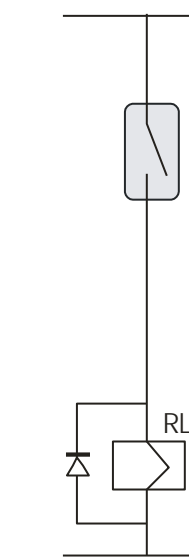
Figura 2. Protección de la bobina en CC
