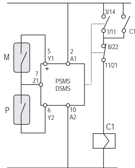
Figura 7. Marcha-Paro con y un relé SMS/DSMS
