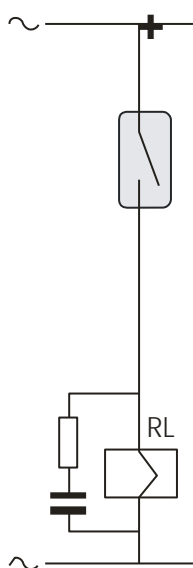
Figura 1. Protección de la bobina en CA CC
