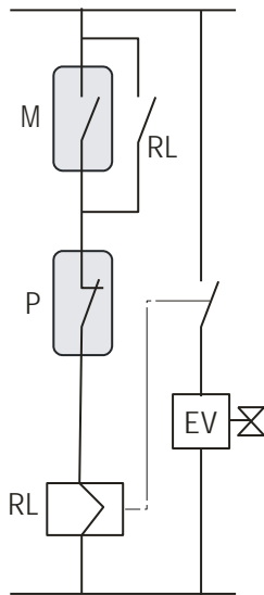
Figura 6. Marcha-Paro con dos contactos dos contactos y un relé auxiliar
