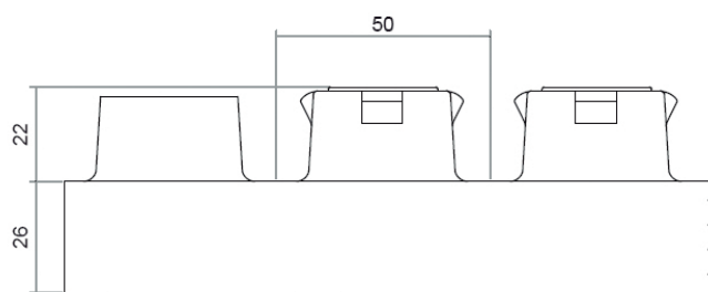
Detalle del perfil (cotas en mm)
