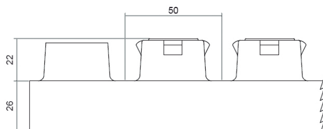
Detalle del perfil (cotas en mm)
