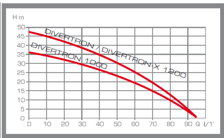
Curva característica 1200
