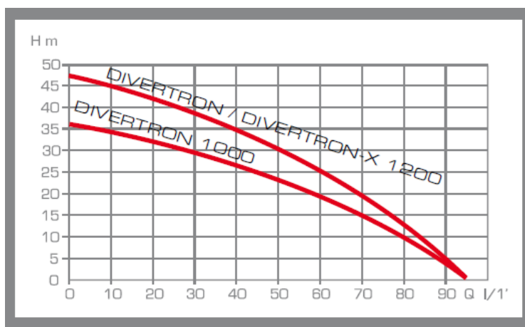
Curva característica 1200
