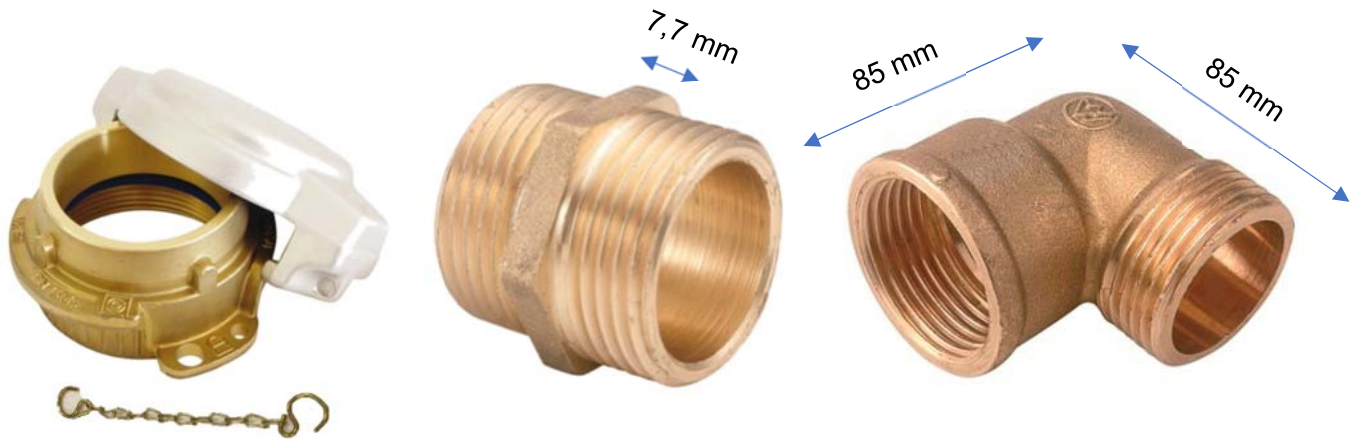
Acople tipo Campsa, cadena y tapa
