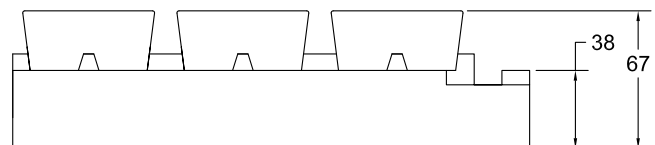
Detalle del perfil (cotas en mm)
