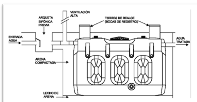
Fig.7 Esquema general de una fosa séptica
