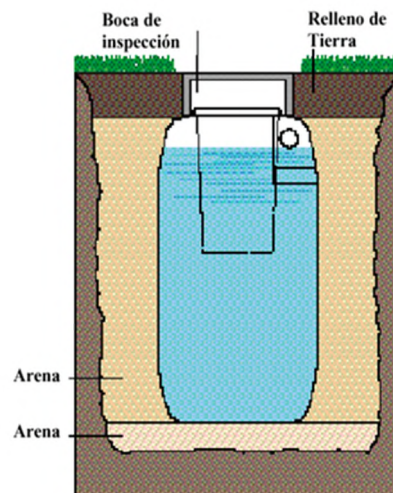
Fig 5. Detalle de zanja con depósito
