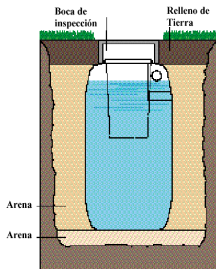
Figura 8 Detalle de zanja con depósito
