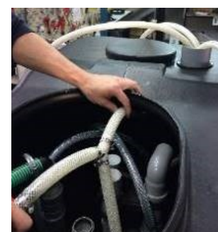
Imagen 10 Unión de las mangueras de los difusores en el depósito digestor, grifo de regulación y salida de mangueras
