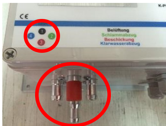
Imagen 11 Entronques para la conexión de las mangueras en el cuadro eléctrico
