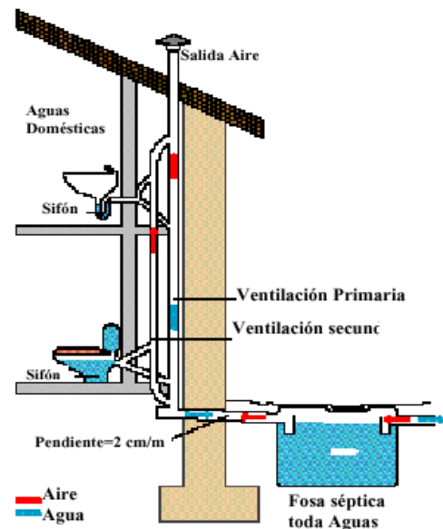
Figura 7 Sistema de aireación
