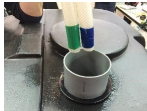
Imagen 1 Sistema Air-Lift (izquierda) y orificio para paso de mangueras (derecha)
